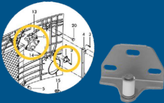
Cód. BL: W50077.4 Cód. Original: 2R2823507 Descrição: Batente do Capô VW Constellation Material: Ferro Cor: Cinza (Natural)
