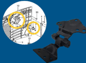
Cód. BL: W50077.2 Cód. Original: 2R2823301 Descrição: Dobradiça do Capô L.E. VW Constellation Cód. BL: W50077.3 Cód. Original: 2R2823302 Descrição: Dobradiça do Capô L.D. VW Constellation Material: Ferro Cor: Preto (Epóxi)
